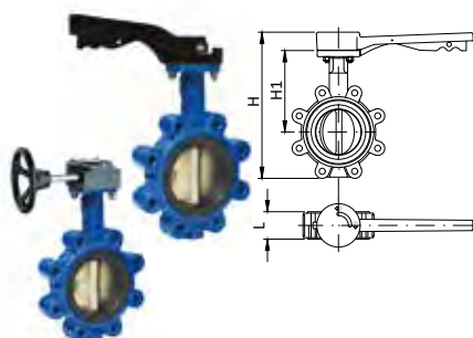
DN 200 FORNITA CON RIDUTTORE
